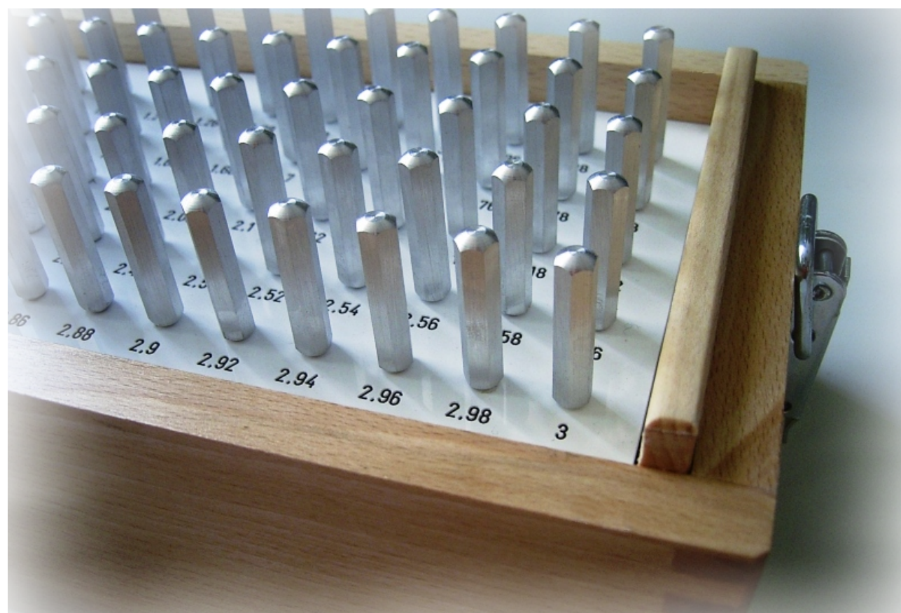
Satz 2-3 mm Ø (101teilig) mit speziellem Holzetui
